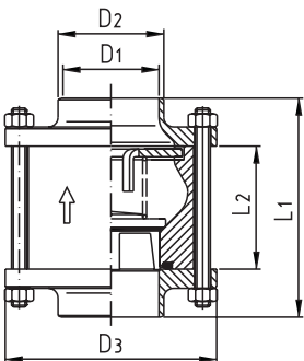
Тарельчатый обратный клапан Zoll для ZFA check valve -Zoll- btw. flangers
