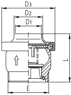
Тарельчатый обратный клапан ДИН GS check valve -DIN- male/welding end
