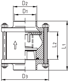
Тарельчатый обратный клапан ДИН для ZFA check valve -DIN- btw. flangers
