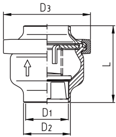
Тарельчатый обратный клапан ДИН SS check valve -DIN-welding ends
