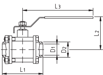
Трехкамерный шариковый кран сварка/сварка port ball valve
