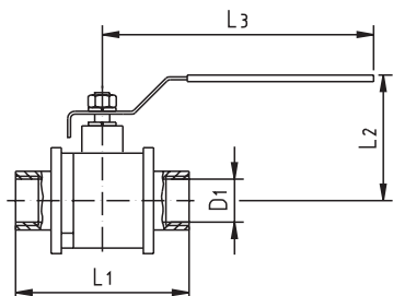
Двухкамерный шариковый кран резьба/резьба port ball valve
