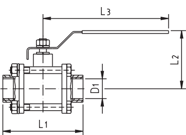
Трехкамерный шариковый кран резьба/резьба port ball valve
