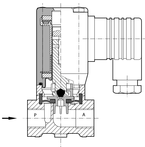
Вид в разрезе GEMÜ 8257
