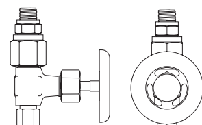
Пробоотборный клапан G 3/8 / Ermeto 8S
