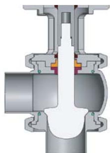
Эквипроцентный затвор
