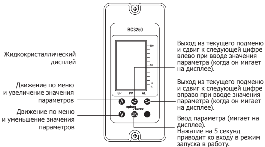
Рис. 1 Передняя панель контроллера и обозначения
