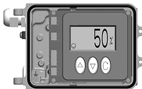
SP400 с открытой крышкой
